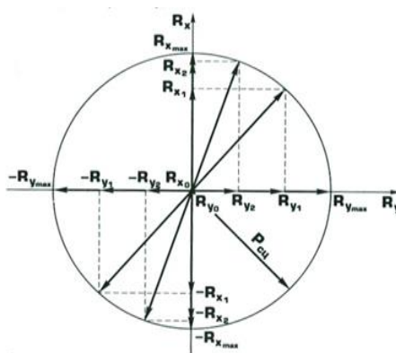
Рис.1. Круг силы сцепления P_{сцл} : сложение продольных R_x и боковых R_y реакций, действующих в пятне контакта колеса с дорогой
